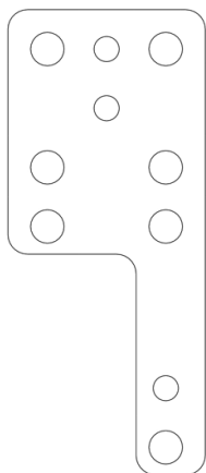
Адаптер ИВЮТ. 741134.018
