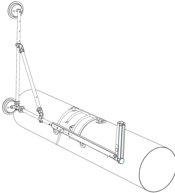
Походное положение
