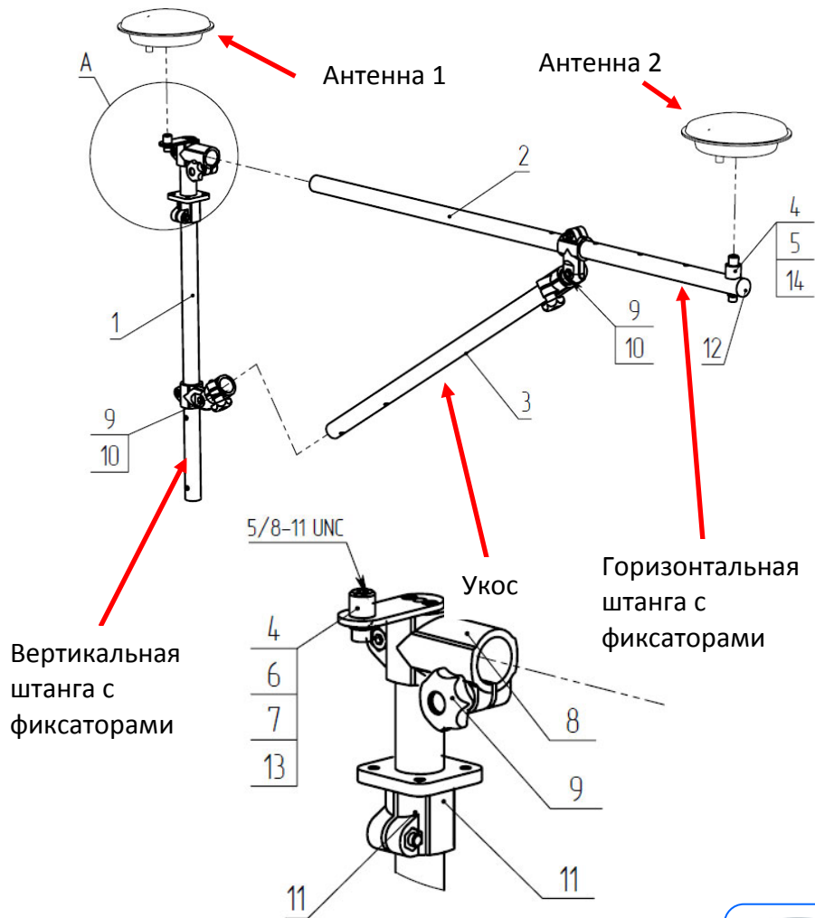
Походное положение
