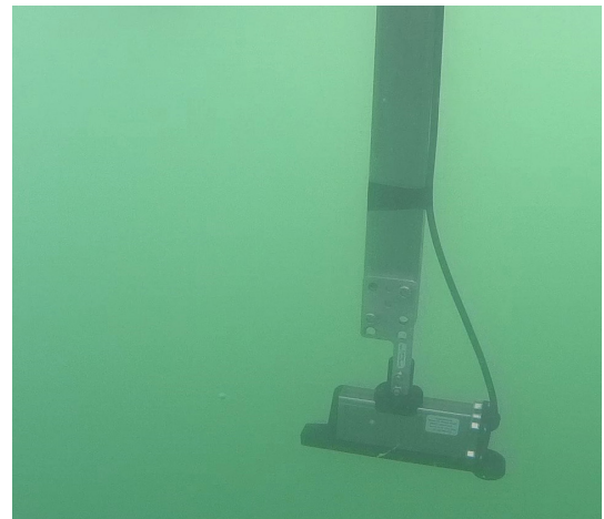
Установка гидролокатора H5s(e)7 на штангу с помощью адаптера ИВЮТ.741134.018
