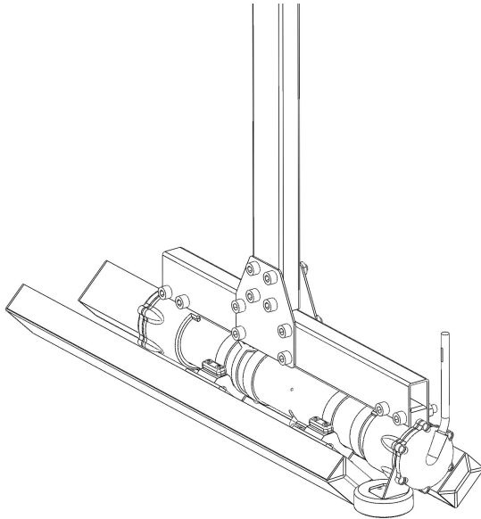
Установка гидролокатора H5s(e)1 на штангу с помощью адаптера ИВЮТ.301529.009
