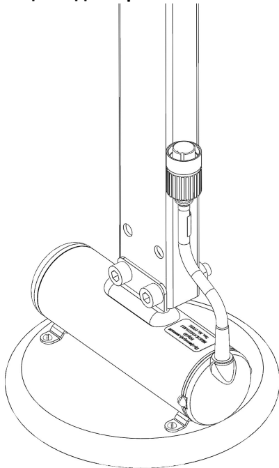
Установка гидролокатора H5s(e)1 на штангу с помощью адаптера ИВЮТ.301529.009
