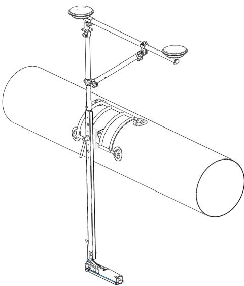
Пример установки набора и комплекта навигации
