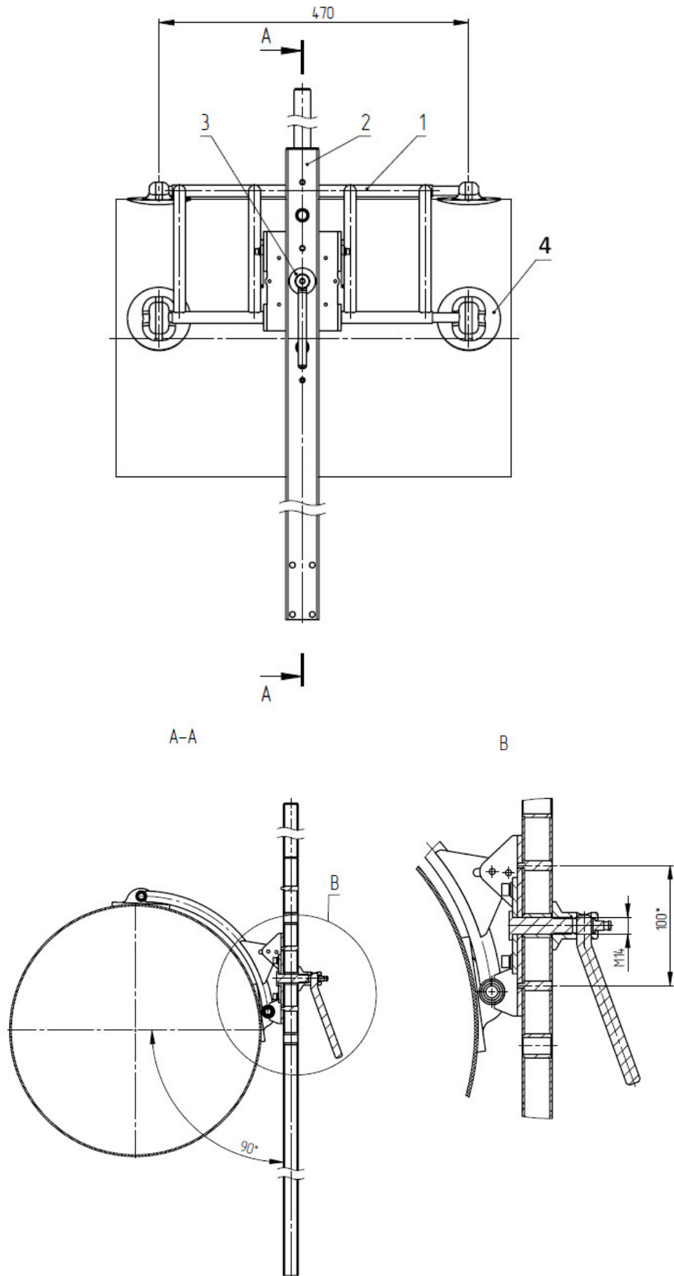
Габаритные и установочные размеры
