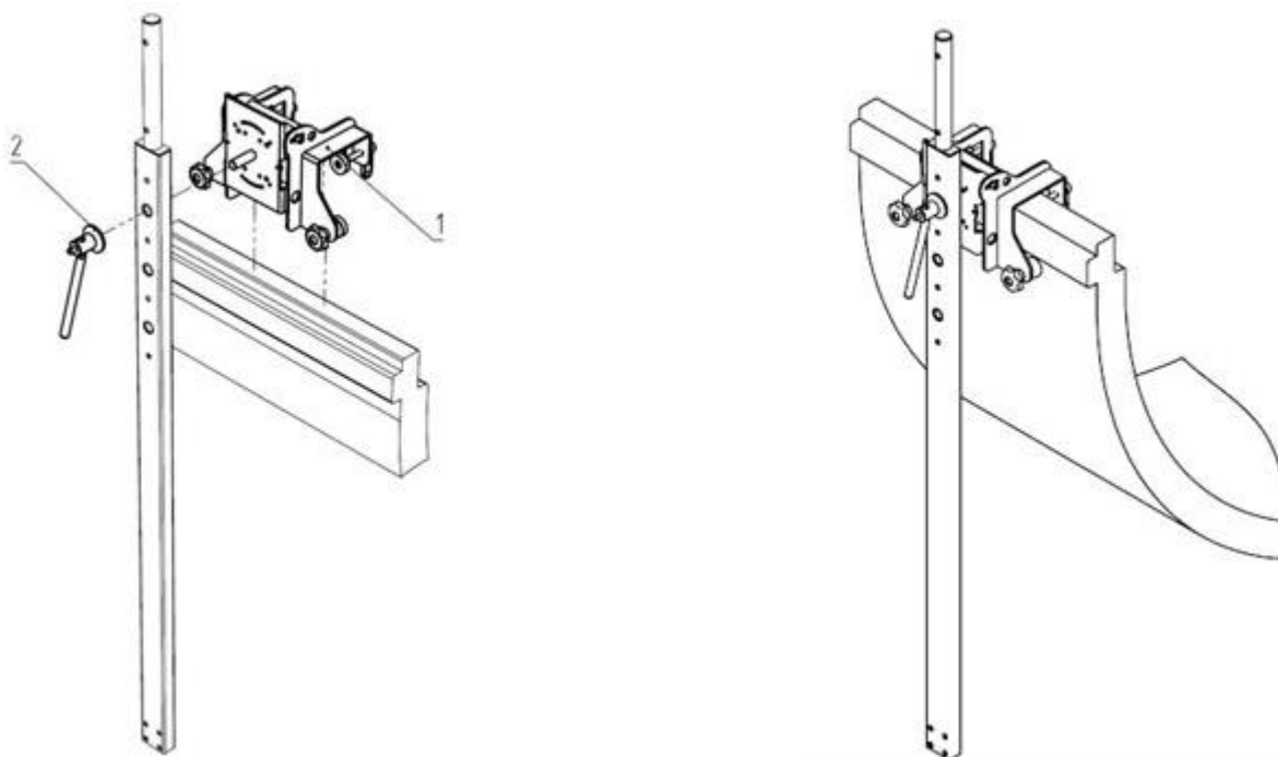
Крепление набора к борту
