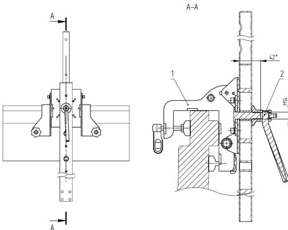
Крепление набора к борту
